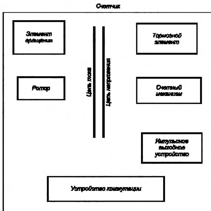
Рисунок С.1 — Структурная схема электромагнитного счетчика
