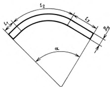
Отвод типа 1
