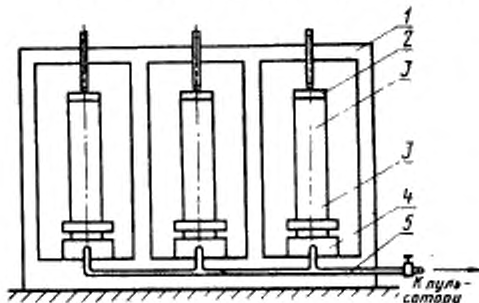
1—рама машины; 2—верхняя винтовая часть оголовка; 3—образец; 4—гидрозомократ; 5—маслопровод.
