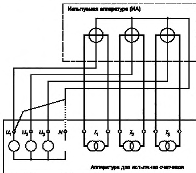
Рисунок С.1 — Схема моделирования состояния замыкания на землю в фазе 1
