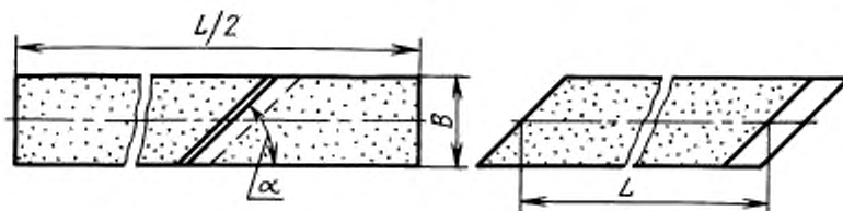
Развертка
