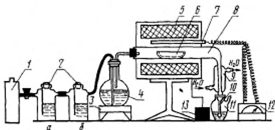
1 — баллон с азотом; 2 — промывные склянки; 3 — электролитка; 4 — паровозобразователь; 5 — трубчатая печь; 6 — кварцевая лодочка; 7 — термометр; 8 — кварцевая трубка; 9 — холодильник; 10 — отводная трубка с барботером; 11 — колба-приемник; 12 — милливольметр; 13 — автографоформатор
