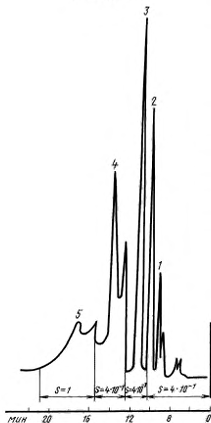
Хроматограмма
