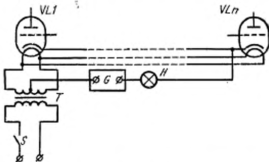
VL1, VLn—испытываемые лампы; T—накальный трансформатор; S—прямая сеть напряжения накала; G—источник питания участка катод-подогреватель; H—сигнальная лампа
