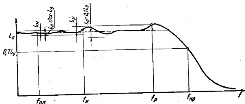
f_{оп} — опорная частота; f_{н} — нормальный диапазон; f_{р} — расширенный диапазон; f_{пр} — верхняя граница полосы пропускания; l_о — значение АЧХ на опорной частоте; l_{н} — абсолютное значение неравномерности в нормальном диапазоне; l_{р} — абсолютное значение неравномерности в расширенном диапазоне; \delta_x — относительная погрешность коэффициента отклонения
