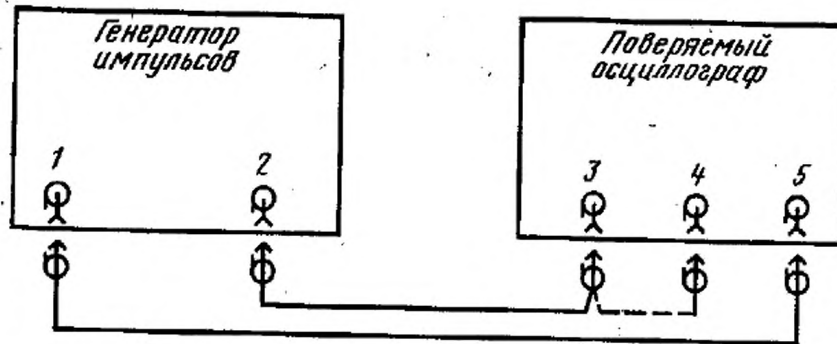
1 — выход синхронизирующих импульсов; 2 — выход основных импульсов; 3 — вход усилителя У; 4 — выход калибратора осциллографа; 5 — вход синхронизации
