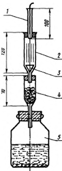
Прибор для определения мышьяка
