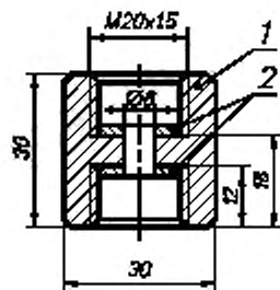
1 — переходник; 2 — прокладка
