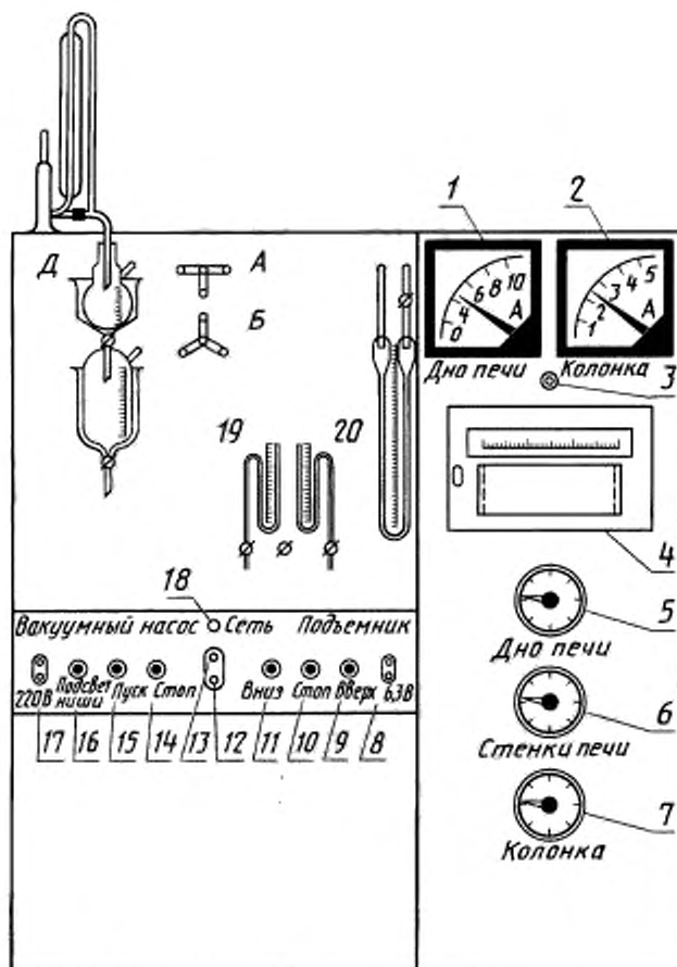
1 — амперметр на 10 А; 2 — амперметр на 5 А; 3 — сигнальная лампа для контроля включения или выключения нагрева стенок печи; 4 — потенциометр автоматический марки ПС1—08 или КСП2—027; 5—7 — автотрансформаторы типа ЛАТР-1; 8 — розетка для нагрева электродвигателя; 9—15 — кнопки управления, 16 — лампа для подсветки ниши; 17 — розетка для включения переносной лампы или для обогрева переходной трубки от крана до приемника; 18 — сигнальная лампа для контроля включения или отключения аппарата от сети; 19, 20 — вакуумметры ртутные
