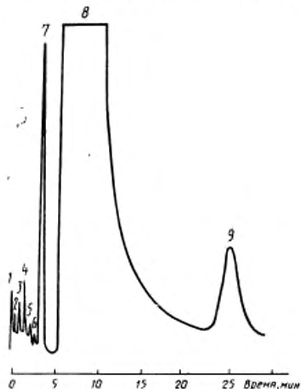
Типовая хроматограмма органических примесей в диэтиленгликоле на колонке с насадкой II
