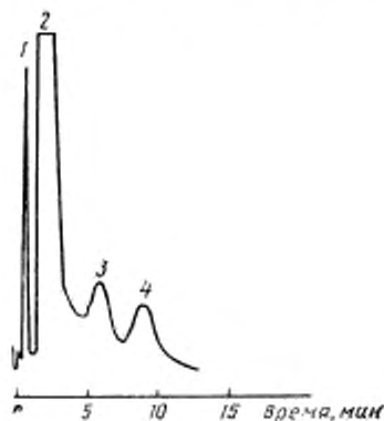
1—углекислый газ; 2—диэтиленгликоль, 3—дециловый спирт; 4—триэтилглицерин
