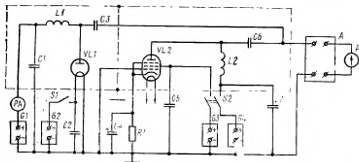
РА — миллиамперметр постоянного тока; G1, G2, G3, G4 — стабилизированные регулируемые источники питания; C1, C2, C4, C5, C7 — развязывающие конденсаторы; C3, C6 — разделительные конденсаторы; L1, L2 — дроссели; S1, S2 — выключатели; VL1 — шумовой диод; VL2 — испытываемая лампа; R1 — резистор; A — избирательный усилитель; P — индикатор
