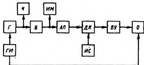
Г—генератор СВЧ; В—ферритный вентиль; АП—переменный прецизионный аттенуатор; ДК—измерительная диодная камера; ВУ—видеоусилитель; О—осциллограф; Ч—частотомер; ИМ—измеритель мощности; ГИ—генератор прямоугольных импульсов; ИС—источник смещения
