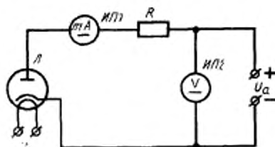
ИП1—миллиамперметр постоянного тока; ИП2—вольтметр постоянного тока; R—резистор, Л—измерительная лампа.
