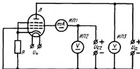
ИП1—миллиамперметр постоянного тока; ИП2, ИП3—вольтметры постоянного тока; R—резистор; Л—жельтываемая лампа.
