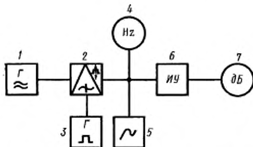
1—звуковой генератор; 2—ключевая схема (импульсный модулятор); 3—генератор прямоугольного напряжения; 4—электро-счетный частотомер; 5—осциллограф; 6—электрическая часть испытываемого ИУ; 7—показывающий прибор ИУ.
