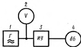
1—звуковой генератор; 2—вольтметр; 3—электрическая часть испытываемого ИУ; 4—показывающий прибор ИУ
