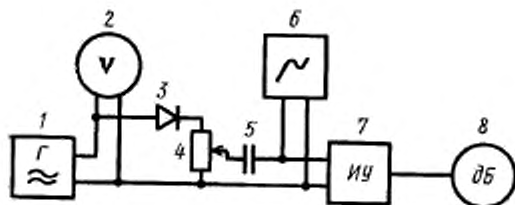
1—звуковой генератор; 2—вольтметр; 3—диод Д 226 (или до соотв.); 4—потенциометр 600 Ом; 5—конденсатор 1 мФ; 6—осциллограф; 7—электрическая часть испытуемого ИУ; 8—показывающий прибор ИУ
