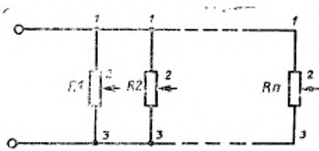
R_1 , R_2 , R_n — испытываемые резисторы, 1, 3 — неподвижные контакты; 2 — подвижный контакт
