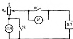
B1 —испытываемый выключатель; B2 —выключатель для защиты амперметра; И —индикатор; ИП —источник питания постоянного или переменного тока; мА —миллиамперметр; R н —нагрузочный резистор
