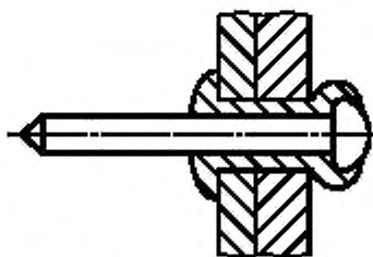
Рисунок 7 — Неразрывающийся вытяжной сердечник
