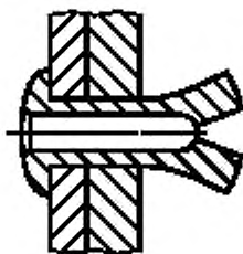
Рисунок 15 — Разделяющийся конец
