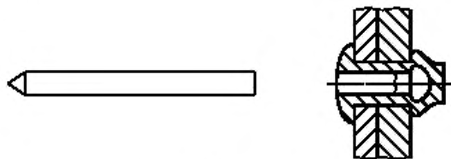
Рисунок 13 — Закрытый конец
