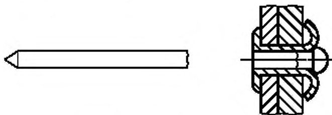
Рисунок 14 — Разделяющийся конец
