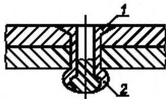
1 — головка «слепой» заклепки; 2 — «слепая» головка
