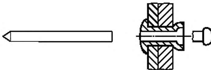
Рисунок 6 — Сердечник с отрывающейся головкой
