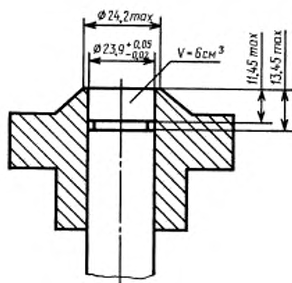
Камера прибора «ухо искусственное»
