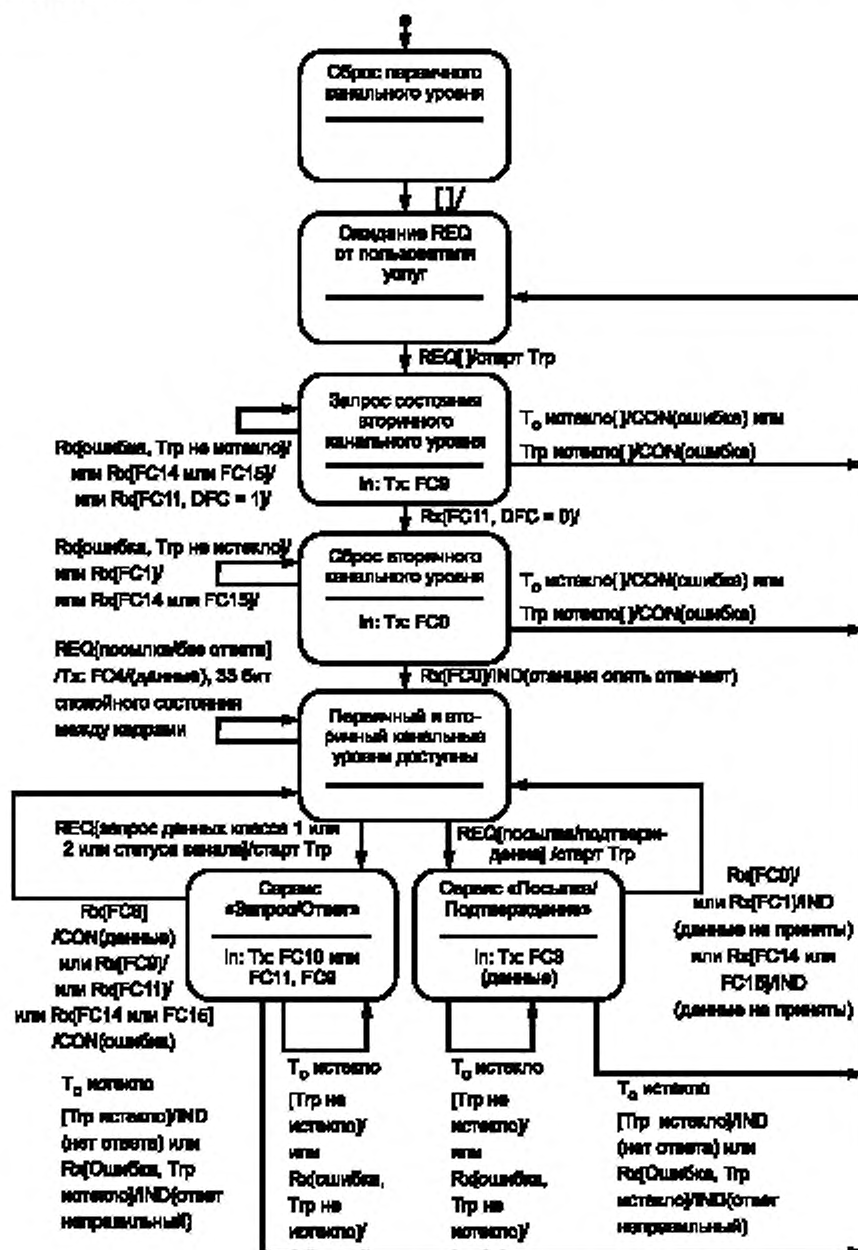
Рисунок 5 — Диаграмма переходов состояний для небалансной передачи: первичный канальный уровень
