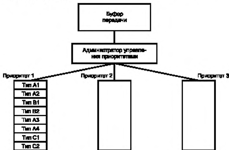
Рисунок 13 — Представление типов объектов информации в приоритетных буферах
