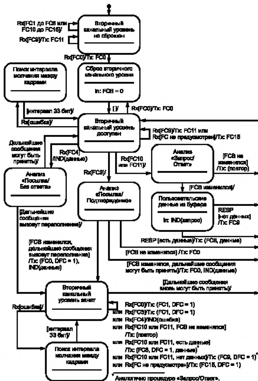
Рисунок 6 — Диаграмма переходов состояний для небалансной передачи: вторичный канальный уровень
