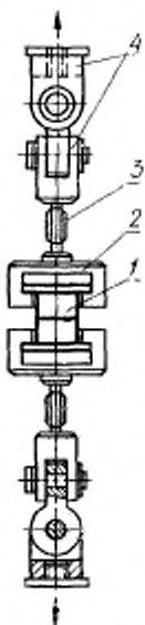
1—образец; 2—захват; 3—тяга; 4—шарнирная подвеска.
