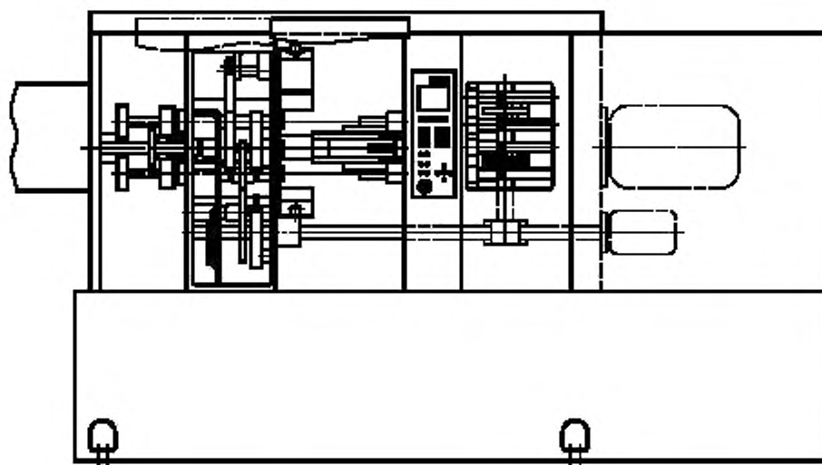
б) Пример многоспindleльного пруткового кулачкового токарного автомата
