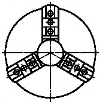
Рисунок 2 — Зажимной патрон
