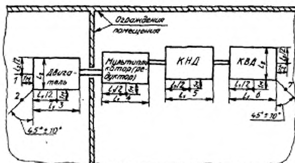
1—7 — точки измерения шума; КНД — корпус высокого давления компрессора; КВД — корпус высокого давления компрессора; l_1 и l_2 — длина и ширина обтекающего источника шума параллелепипеда
