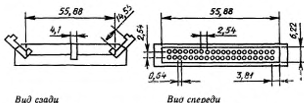
Розетка одностороннего интерфейсного соединителя
