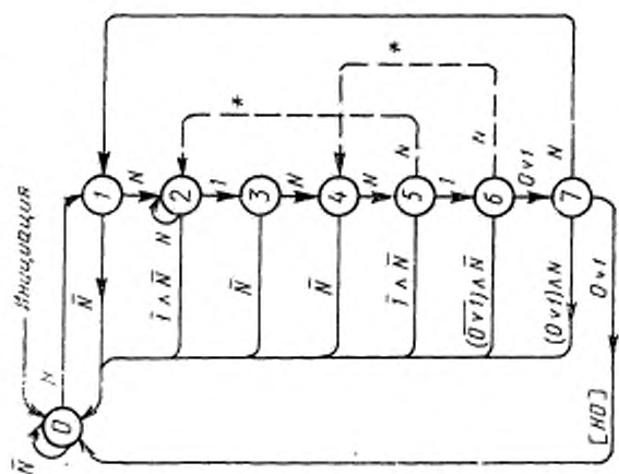
Конечный автомат обнаружения ОК
