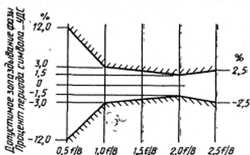
ЧАСТОТА ПЕРЕДАЧИ СИГНАЛОВ* Период символа — УДС
