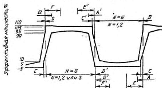
Форма оптического волнового сигнала
