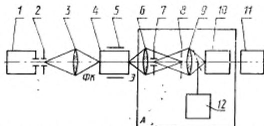
1 — осветитель; 2 — диафрагма со щелью; 3 — входная оптика (микрообъектив в обратном ходе); 4 — ЭОП; 5 — держатель ЭОП; 6 — выходной микрообъектив; 7 — выходной экран микрообъектива; 8 — анализирующий растр; 9 — коллектив; 10 — приемник излучения; 11 — регистрирующее устройство; 12 — микроскоп; ФК — фотокатод; Э — экран; А — анализирующий блок
