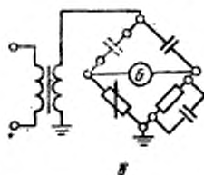
Схема с заземленной диагональю
