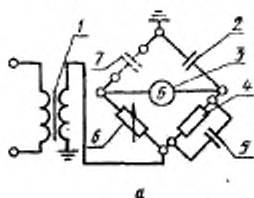
Схема с заземленной диагональю
