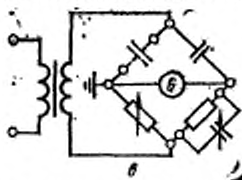
Схема с заземленной диагональю
