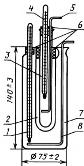
Схема прибора для определения температуры кристаллизации
