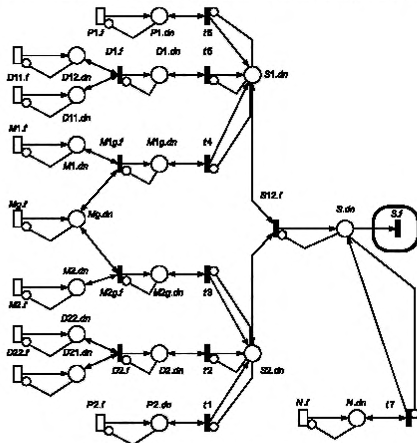
Рисунок А.9 — Сеть Петри мультипроцессорной системы
