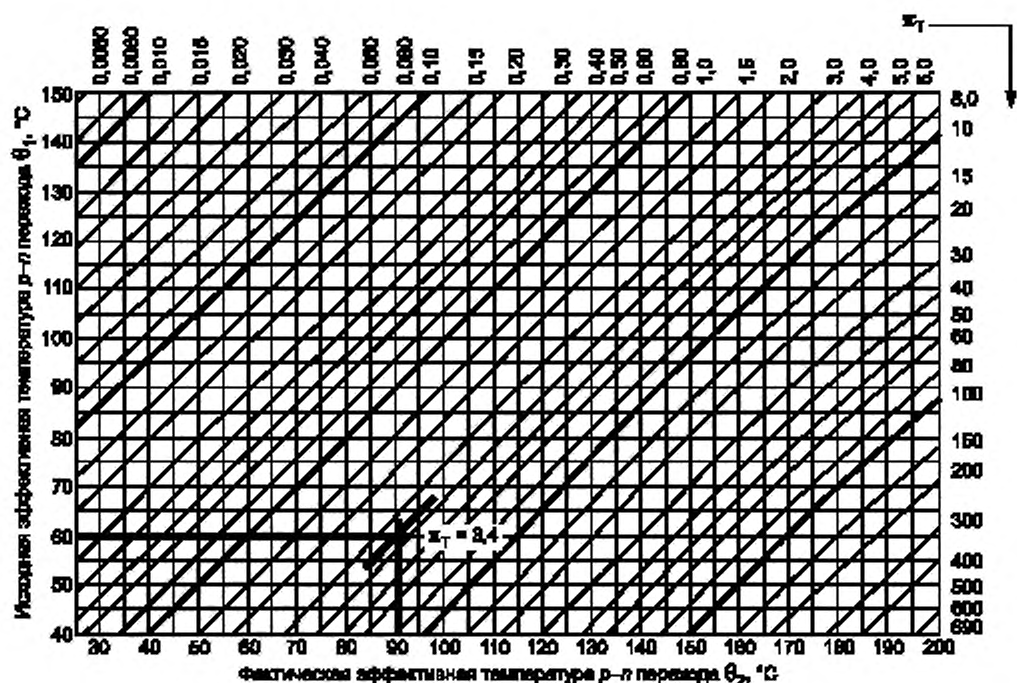
Рисунок А.1 — Зависимость интенсивности отказов от температуры
