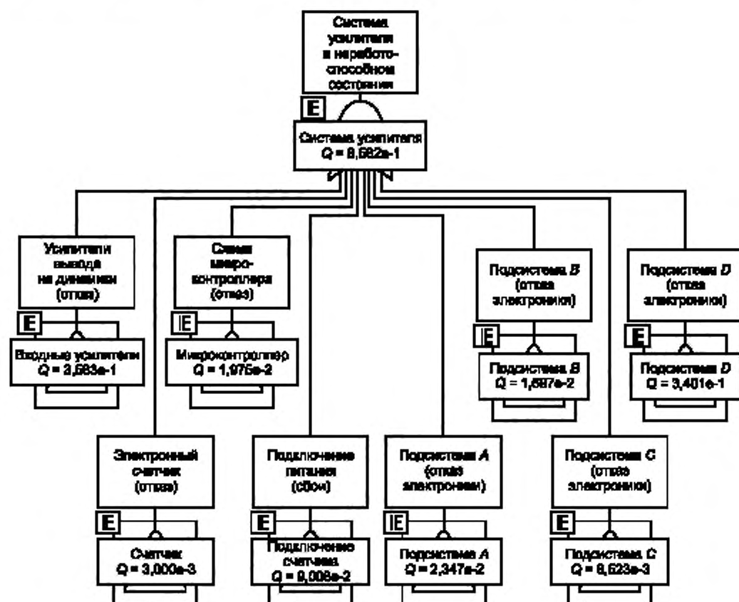
Рисунок А.2 — Дерево неисправностей для аудиоусилителя
