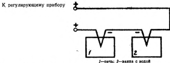
Схема соединения термопреобразователей
