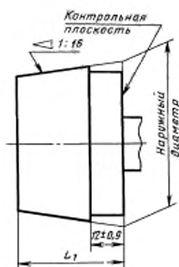
Калибр-пробка Г
