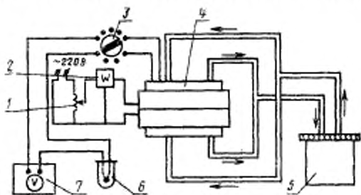
1—автотрансформатор; 2—ваттметр; 3—переключатель термомаяр; 4—рабочая часть; 5—термостат; 6—холодный спай термопар; 7—электроцифровой вольтметр
