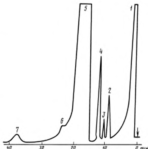
1 — хлороформ; 2 — трифторацетианид + 2-хлортрифторацетианид; 3 — неидентифицированная примесь; 4 — нитробензол; 5 — 2-метокситрифторацетианид; 6 — 3-хлортрифторацетианид + 4-хлортрифторацетианид; 7 — 4-метокситрифторацетианид
