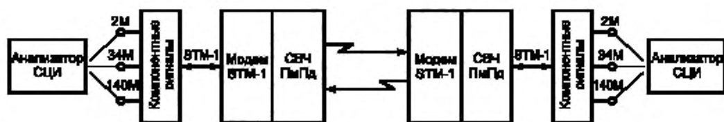
Рисунок 4.3 — Схема измерений показателей качества по ошибкам для ВОЛС
