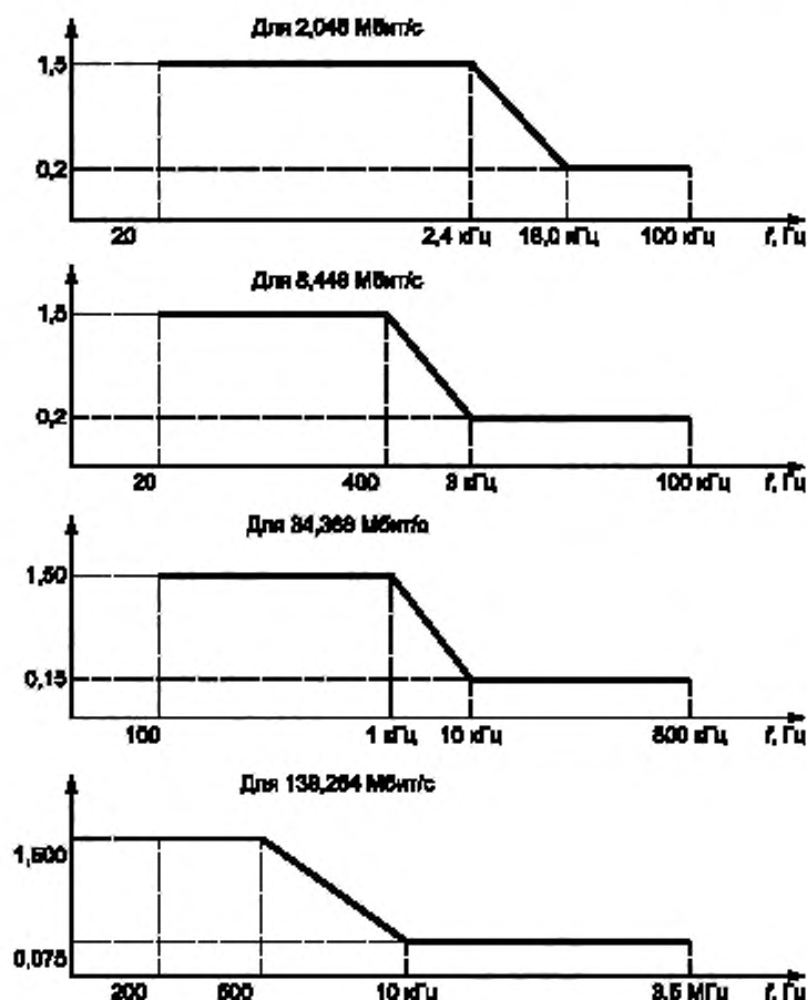
Рисунок 4.16 — Маски сигналов с предельным фазовым дрожанием
