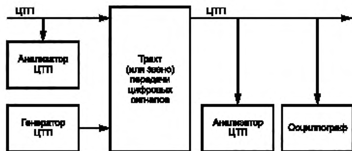
Рисунок 5.1 — Схема проведения измерений параметров цифрового транспортного потока
