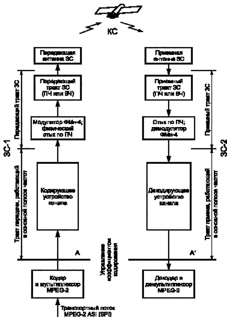
Рисунок 4.10 — Структурная схема СЛТ передачи сигналов ЦТВ
