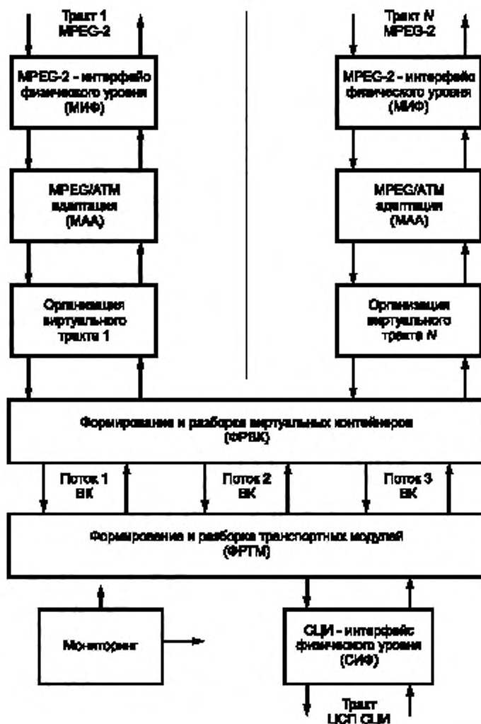
Рисунок 4.2 — Функциональная архитектура аппаратуры преобразования MPEG → СЦИ и СЦИ → MPEG
