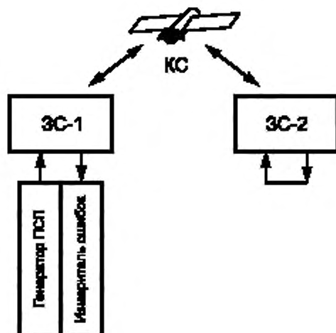
Рисунок 4.13 — Измерение показателей качества с включением шлейфа
