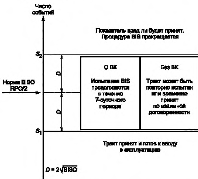
Рисунок 4.14 — Схема процедуры принятия решения о вводе в эксплуатацию
