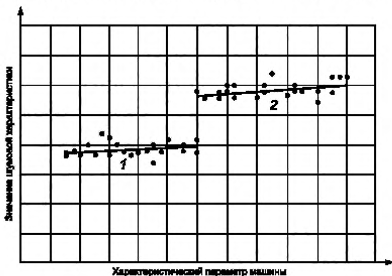
Рисунок В.1 — Разделение данных на две группы
