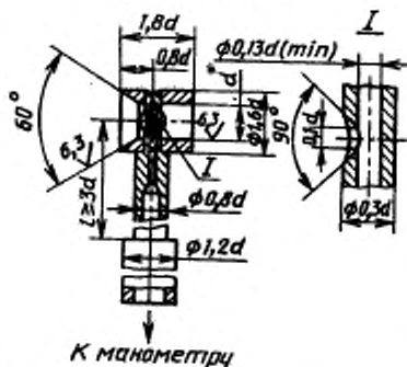
Основные размеры приемной части приемника полного давления
