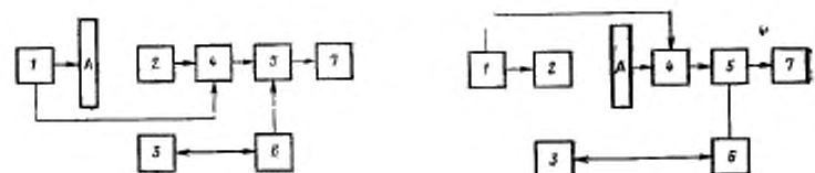
а. Испытуемая антенна в передающем режиме
