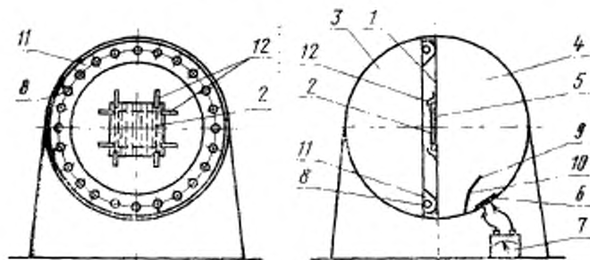
Схема диффузомера
