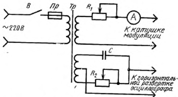
B—выключатель; Pr—предохранитель; R 1 —регулируемый резистор; R 2 —резистор регулировки фаз; C—конденсатор; Tr—трансформатор
