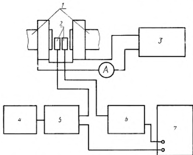
1—полюсные наконечники; 2—первичные измерительные преобразователи; 3—источник модулирующего напряжения и фазоинвертер; 4—частотомер; 5—образцовый измеритель магнитной индукции; 6—поверяемый Тесламетр; 7—двухлучевой осциллограф
