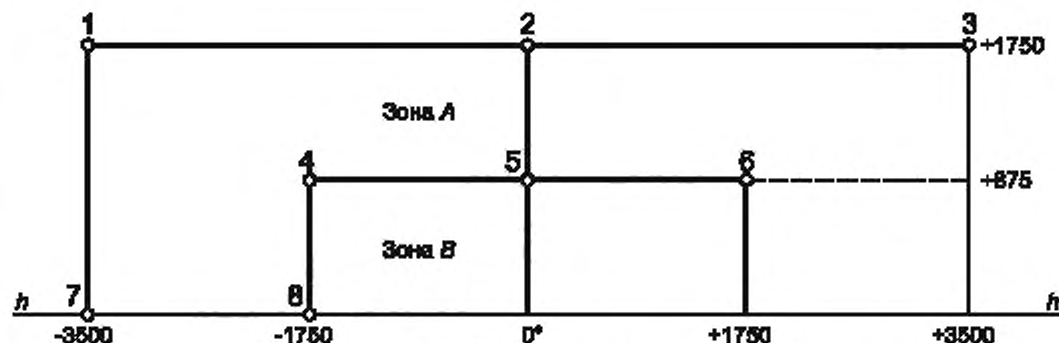
Рисунок 2 — Точки измерения
