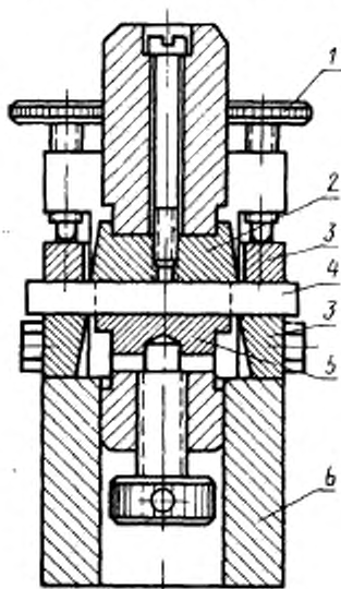
1 — винт; 2 — нож; 3 — опоры; 4 — образец; 3 — опорная плита; 6 — корпус
