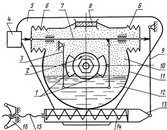
1 — неподвижные образцы-колодки; 2 — подвижный образец-ролик; 3 — рычажный многозвенник; 4 — износоизмеритель; 5 — стойка корпуса (корпус не показан); 6 — герметизирующие сильфоны; 7 — шток; 8 — смотровое стекло; 9 — рычаг; 10 — хладагент; 11 — камера; 12 — маслохладоновая смесь; 13 — корпус нагружающего устройства; 14 — пружина; 15 — винт; 16 — гайка
