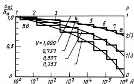
Биномиальное распределение (BB)
