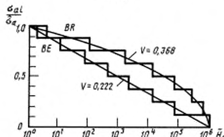
Распределения Рэлея (BR) и экспоненциальное (BE)
