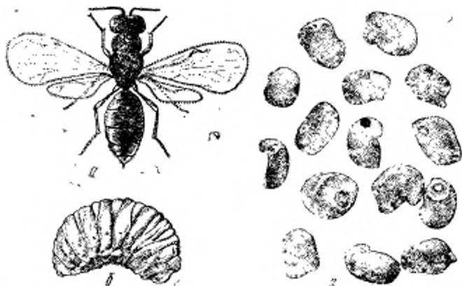
Рис. 8. Акациевый семяед (толстоножка) ( Eurytoma saganae Nik.): а—взрослое насекомое; б—личинка, в—поврежденные семена.
