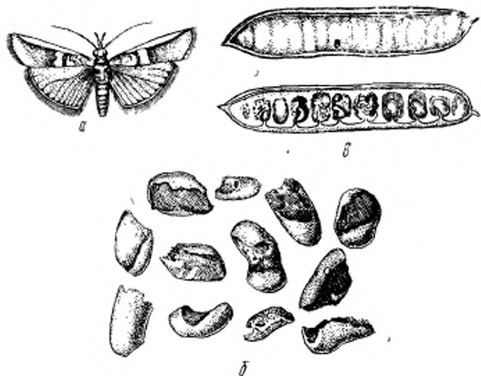
Рис. 6. Акациевая огневка ( Etiella zinckenella Tr.):
