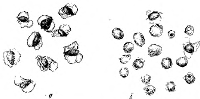
Рис. 12. Березовая галлица-семяд (Semiudobia betulae Winn.);
