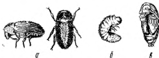
Рис. 19. Хлебный точильщик ( Stegobium raniceum L.):
