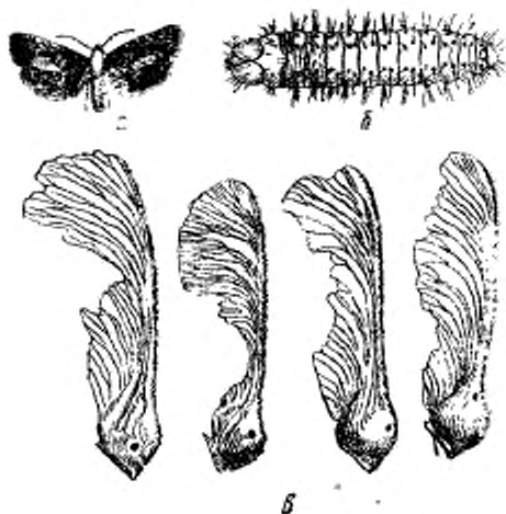
Рис. 10. Кленовая листовертка ( Raminia regiana L.):
