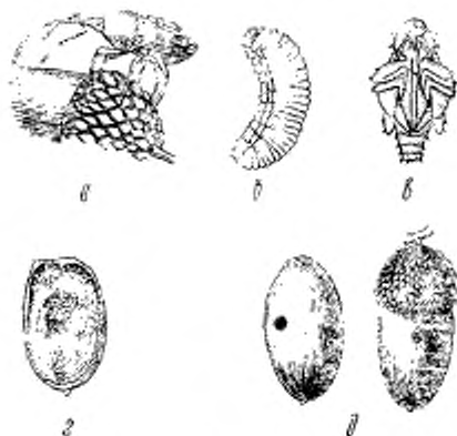
Рис. 15. Желудевый долгоносик ( Balaninus glandium March.):
