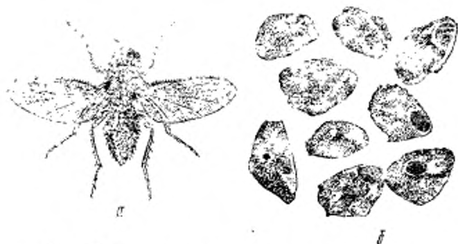
Рис. 3. Лиственничная муха ( Chortophila laricicola Karl.): а—взрослое насекомое; б—поврежденные семена.
