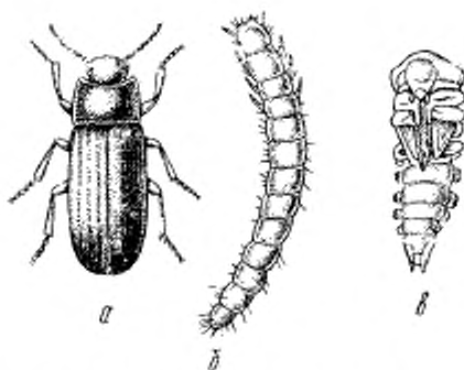
Рис. 21 Большой мучной хрущак ( Tenebrio molitor L.): а—жук; б—личинка; в—куколка.
