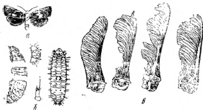
Рис. 9. Кленовая листовертка ( Crobulothra inquinatana Hb.): а—бабочка; б—гусеница; в—поврежденные семена.
