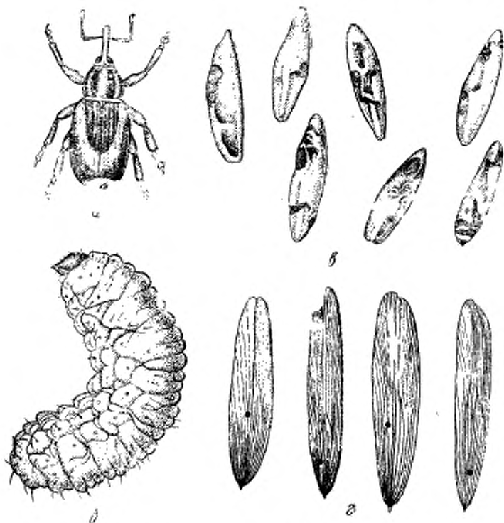
Рис. 13. Ясневый долгоносик-семяед ( Lignyodes enucleator Ranz.): а—жук; б—личинка, в—поврежденные семена; г—крылатки с выходным отверстием личинки.
