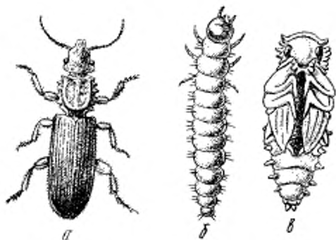
Рис. 22 Суринамский мукоед ( Oryzaephilus surinamensis (L.)). а—жук; б—личинка; в—куколка.
