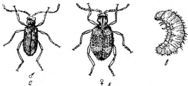
Рис. 18. Вор-притворяжка ( Ptinus fur L.):
