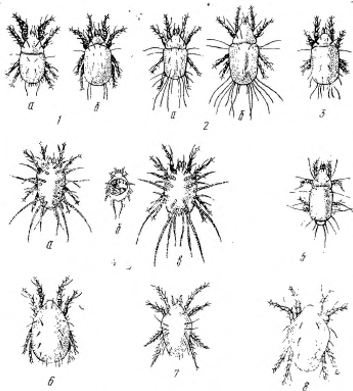
Рис. 23. Разные виды клещей и гипопусов:
