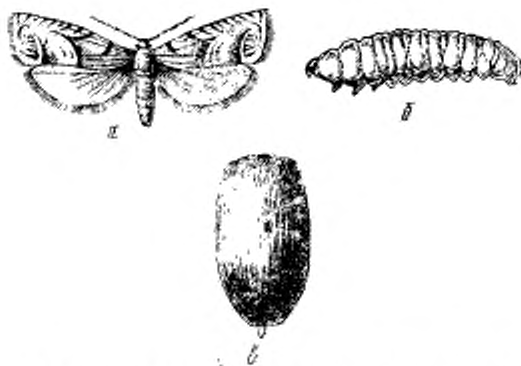
Рис. 16. Желудевая плодожорка ( Carpocarya splendana Нв.):
