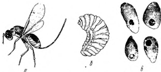
Рис. 4. Еловый короткохвостый сееед ( Megastigmus abietis Seitn.): а—взрослое насекомое; б—личинка; в—поврежденные семена с летними отверстиями насекомого.
