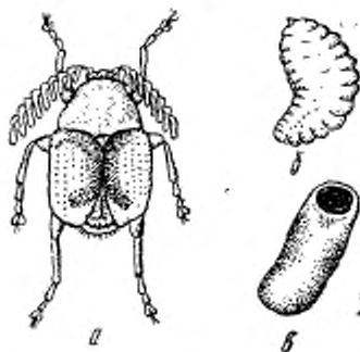
Рис. 7. Акациевая зерновка ( Kitorrhinus quadriplagiatus Mots.):
