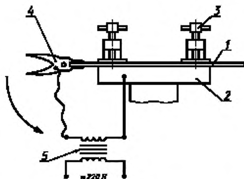
1 — образец проволоки; 2 — токопроводящий стол; 3 — винт прижима; 4 — пассаж; 5 — понижающий трансформатор
