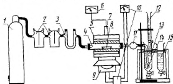
1 — кислородный баллон; 2 — промывные силикаты; 3 — U-образная трубка; 4 — фарфоровая трубка; 5 — трубчатая печь; 6 — гальванометр; 7 — термопара; 8 — фарфоровая лодочка; 9 — терморегулятор; 10 — автотрансформатор с вольтметром; 11 — стеклянный шарик; 12 — микробюретка; 13 — поглотительный сосуд; 14 — барботер; 15 — сосуд с раствором сравнения
