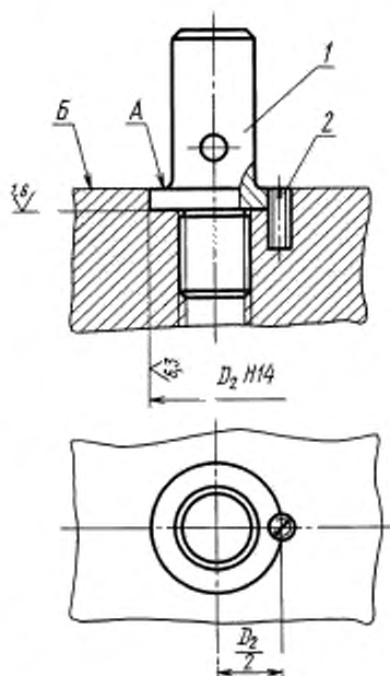
1 — хвостовик; 2 — винт В.М6—8g × 14.14Н по ГОСТ 1477—93
