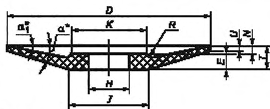
Рисунок 11 — Круги типа 14
