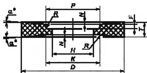
Рисунок 17 — Круги типа 25
