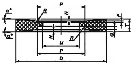
Рисунок 18 — Круги типа 26
