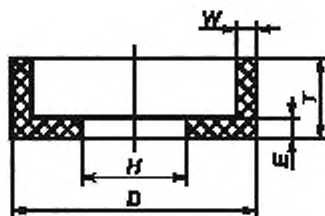
Рисунок 6 — Круги типа 6
