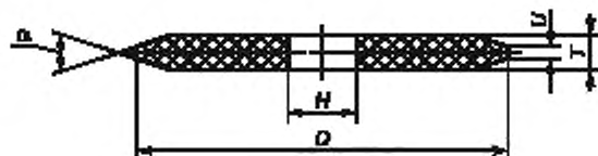
Рисунок 4 — Круги типа 4
