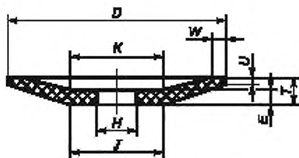
Рисунок 10 — Круги типа 12
