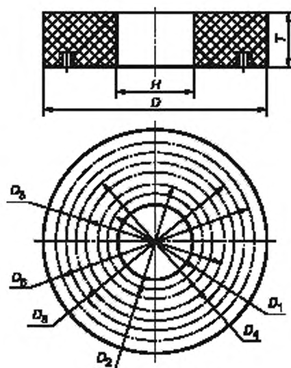
Рисунок 20 — Круги типа 36
