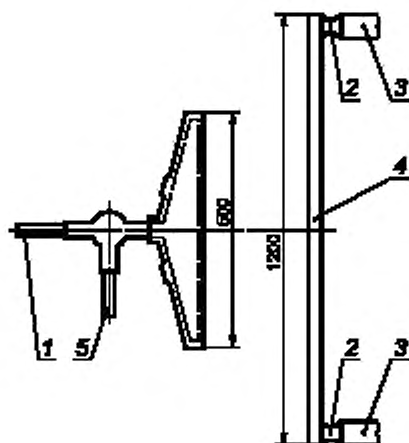
Рисунок 2 — Испытательное устройство (вид сверху)
