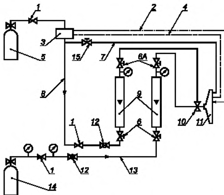
1 — регулятор; 2 — пьезоэлектрический воспламенитель; 3 — устройство для прерывания работы горелки; 4 — контрольные термомпары; 5 — баллон с пропаном; 6 — винтовой клапан (6А — альтернативное расположение); 7 — вспомогательное питание; 8 — поступление газа; 9 — расходомеры; 10 — смеситель Вентури; 11 — горелка; 12 — шаровый клапан; 13 — система подачи воздуха; 14 — баллон со сжатым воздухом; 15 — винтовой клапан на вспомогательном питании
