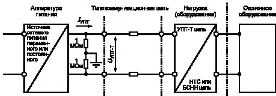
Рисунок А.1 — Пример УПТ-Т системы удаленного электропитания
