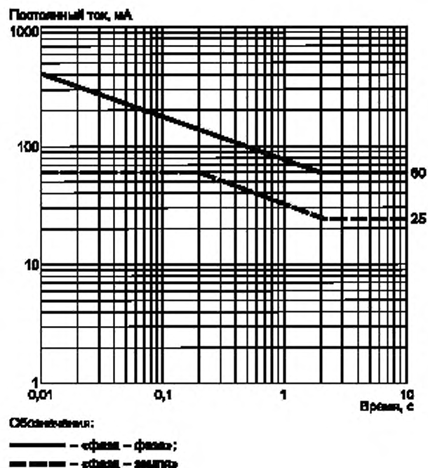
Рисунок 1 — Максимальный ток после единичной неисправности
