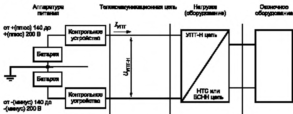
Рисунок А.2 — Пример УПТ-Н системы удаленного электропитания
